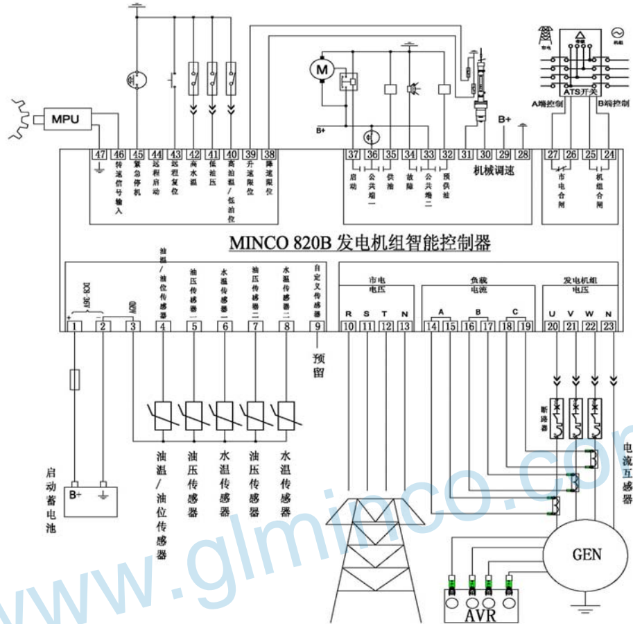
Minco 820B外部接线图（机械调速）
