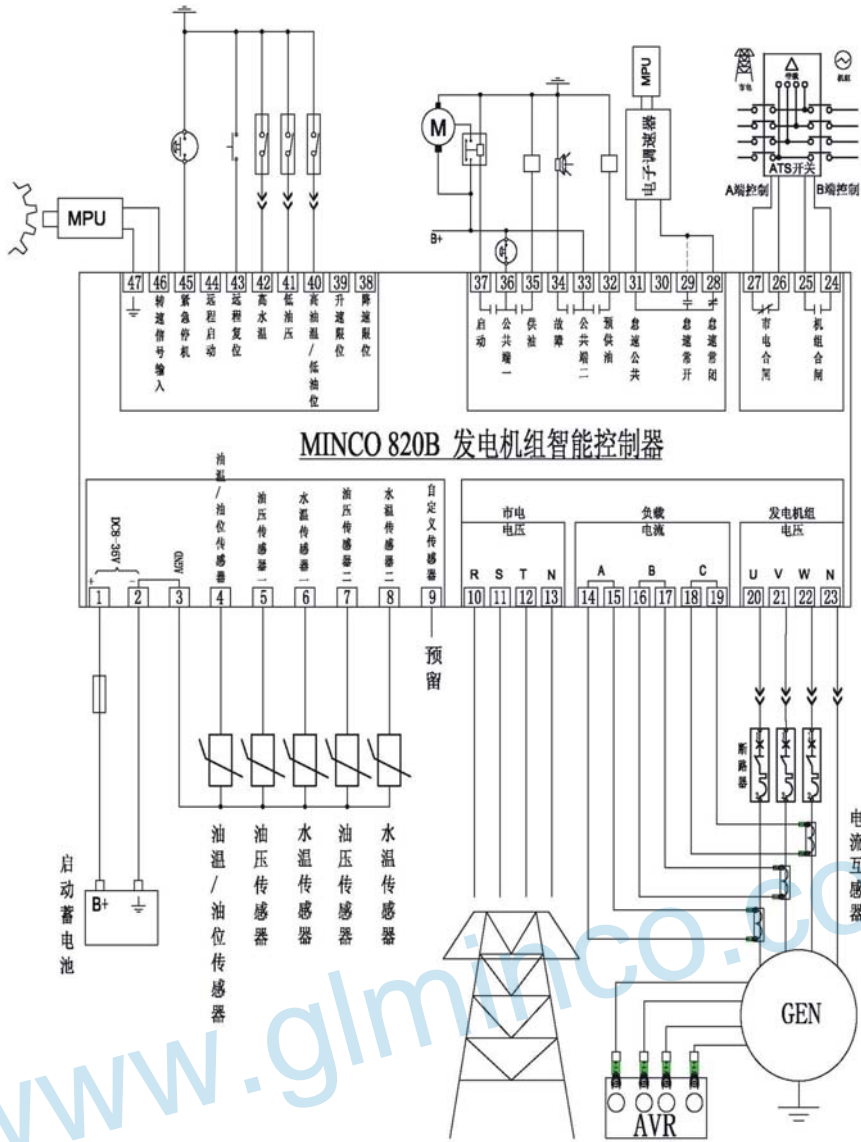
Minco 820B外部接线图 (电子调速)
