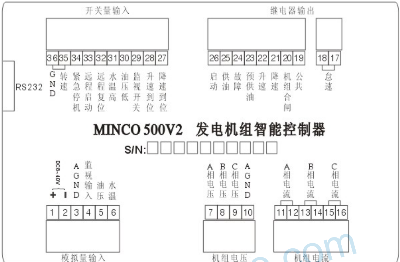
附 3: MINCO 500V2 控制器背面板中英文对照图
