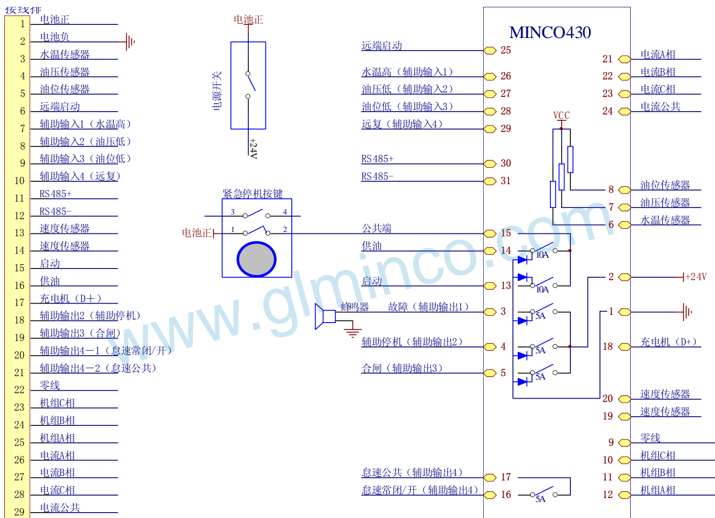
MH4000(MINCO430)控制柜接线图
